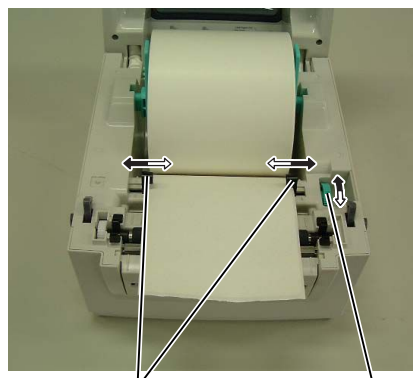
Materialzentrierung Zentrierrad
